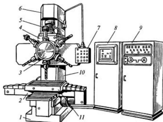
Расположение основных узлов станка 2р135ф2
